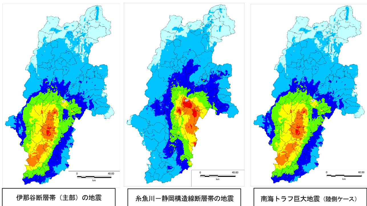
各種地震の地表震度分布
