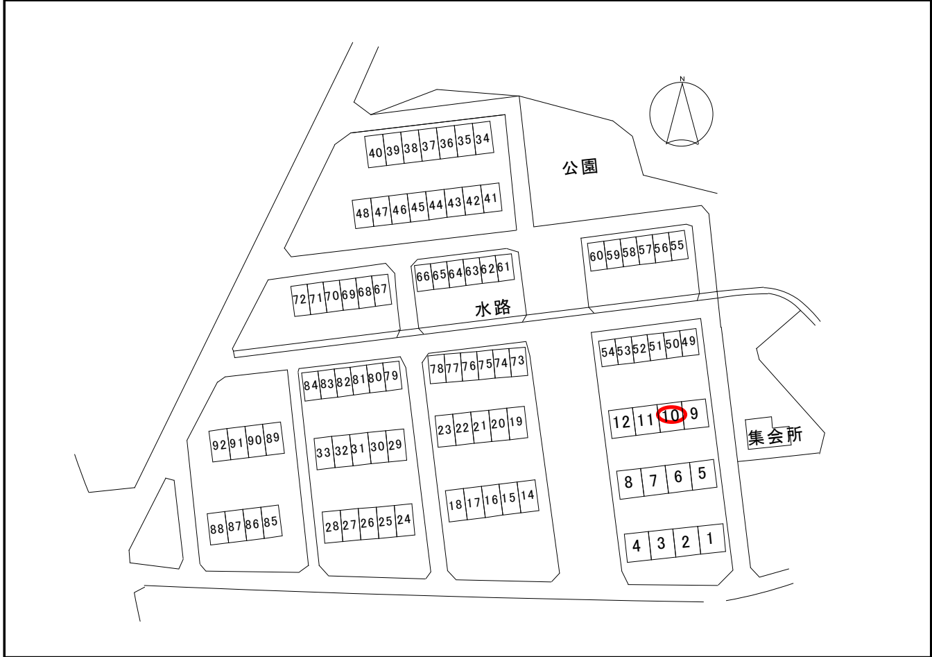
配置図
