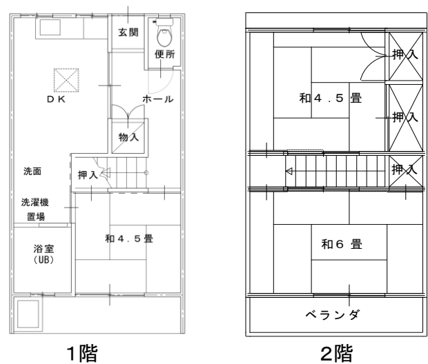
平面図
