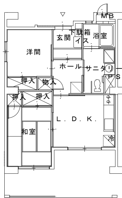
平面図
