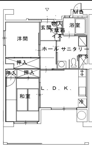
平面図
